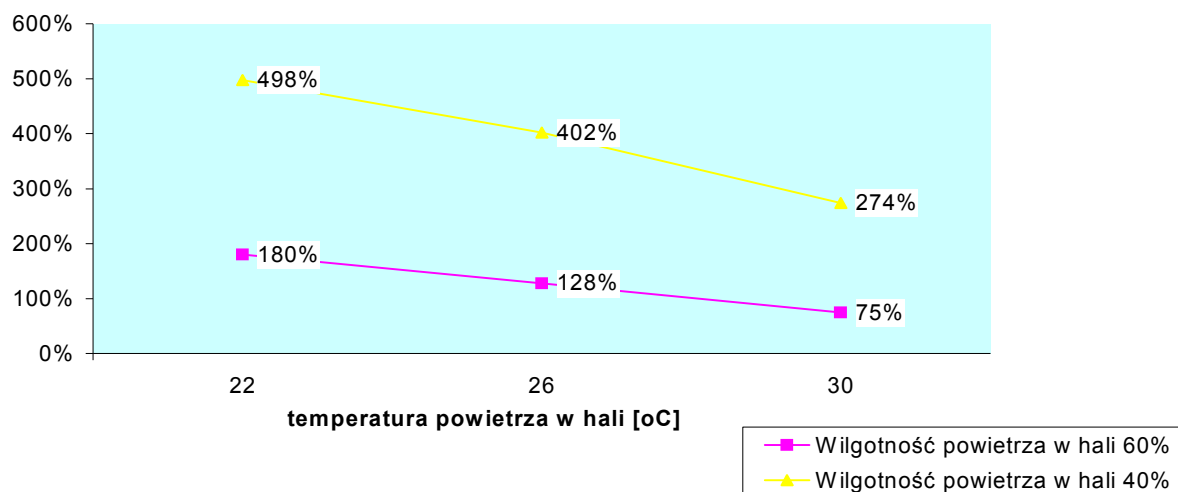
Procentowe zużycie energii na osuszanie dla różnych parametrów powietrza w hali w odniesieniu do zużycia energii przy zalecanej temperaturze 30°C i wilgotności 55%
